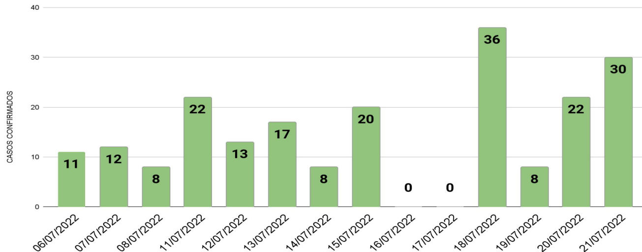
MÉDIA MÓVEL
